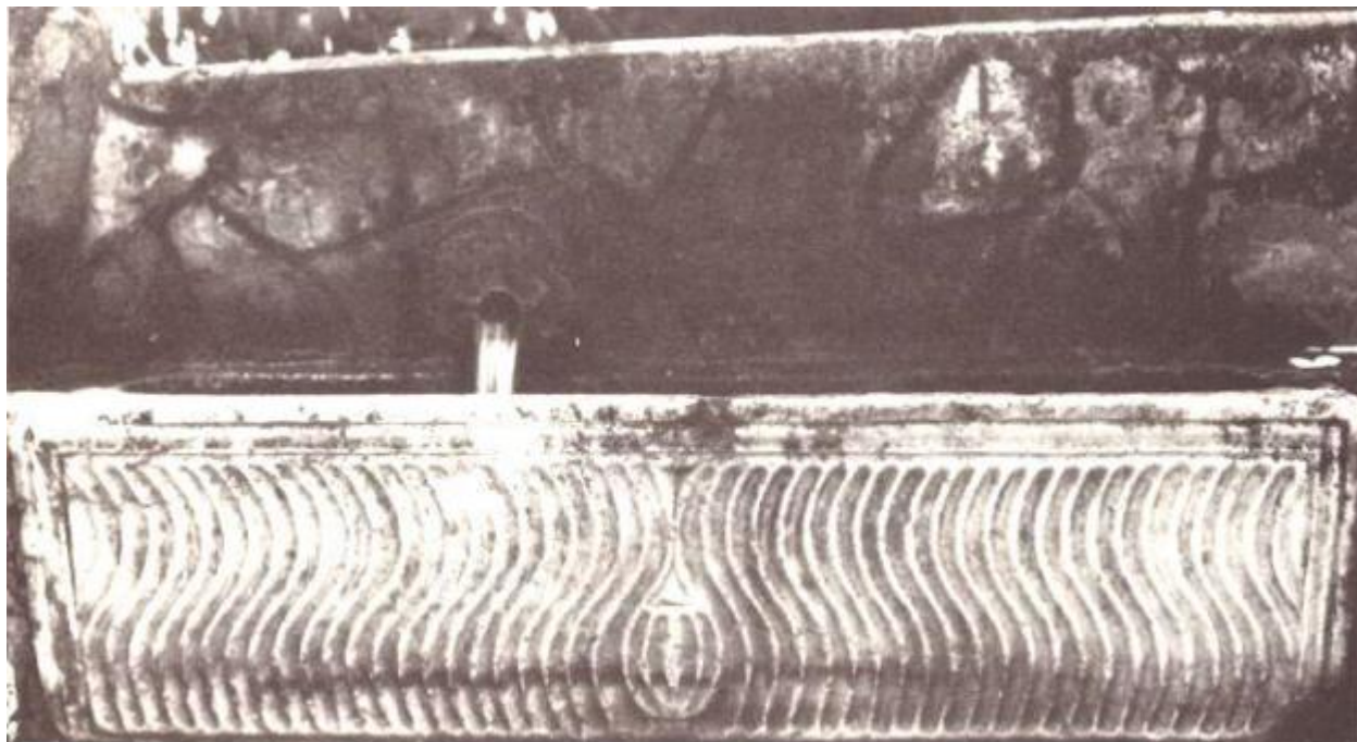
Fig. 6 - Sarcofago strigliato utilizzato come fontana (Zucca 1988, fig. 18).
