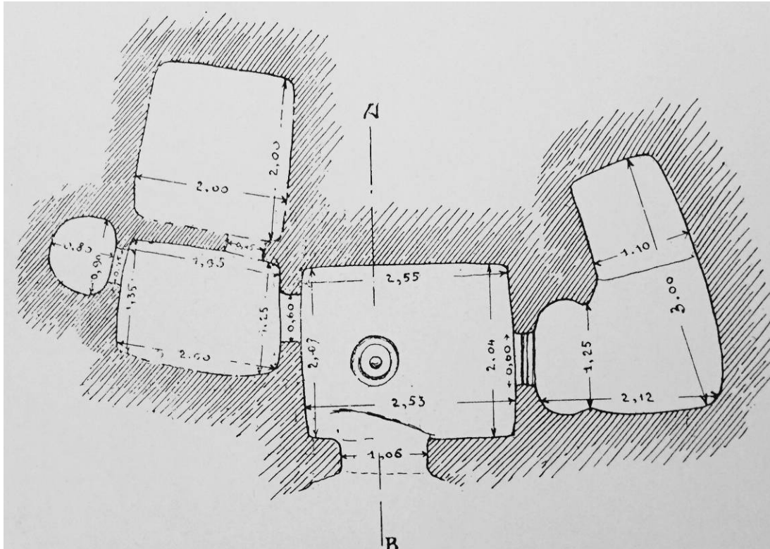
Fig. 3 - Planimetria della domus de janas XIII (da TARAMELLI 1919, fig. 57, pp. 119, 120).
