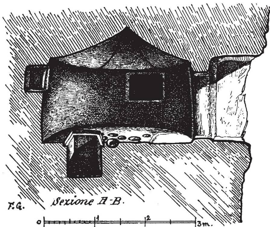
Fig. 3 - Sezione trasversale dell'ipogeo (da TARAMELLI 1919, fig. 45, p. 103).
