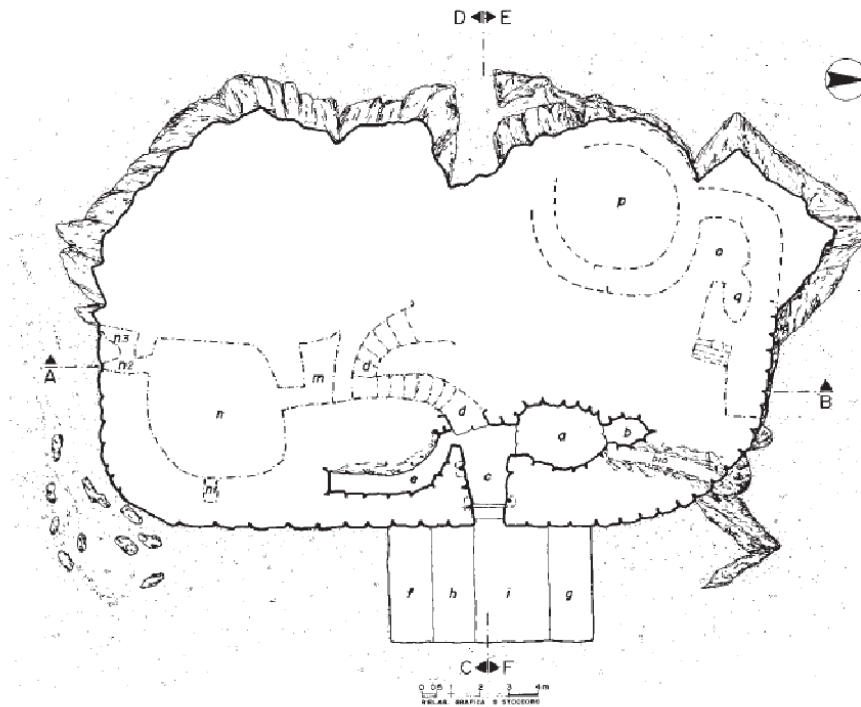
Fig. 1 - Nuraghe Albucciu, planimetria del piano terra (da ANTONA RUJU, FERRARESE CERUTI 1992, fig. 12).
