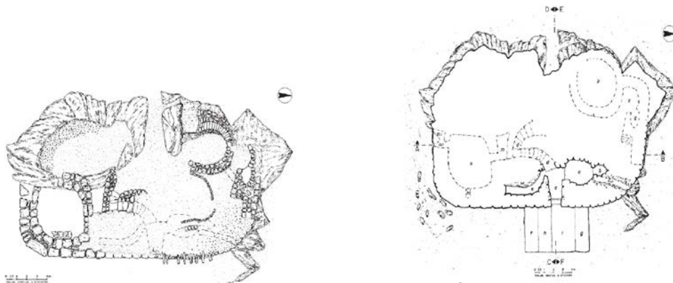
Fig. 1 - Nuraghe Albucciu, planimetria del piano terra e del piano superiore (da ANTONA RUJU, FERRARESE CERUTI 1992, fig. 12).
