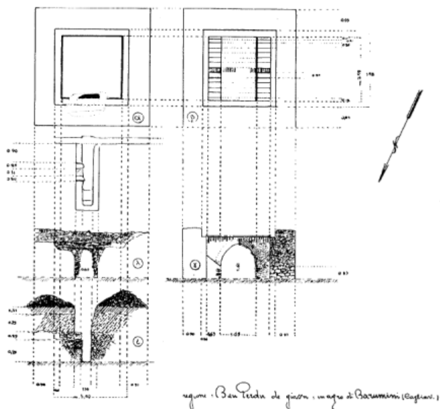
Fig. 3 - Barumini, villa rustica di Età Romana in località Bau Pardu di Sotto (da Lilliu 1940, fig. 4, p. 379).
