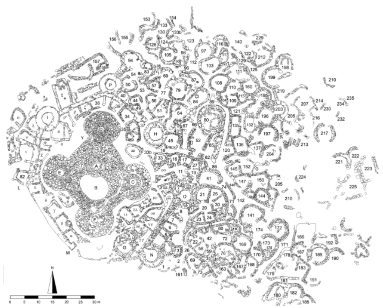
Fig. 1 - Planimetria del sito di Su Nuraxi (da Paglietti 2013, fig. 6, p. 64).
