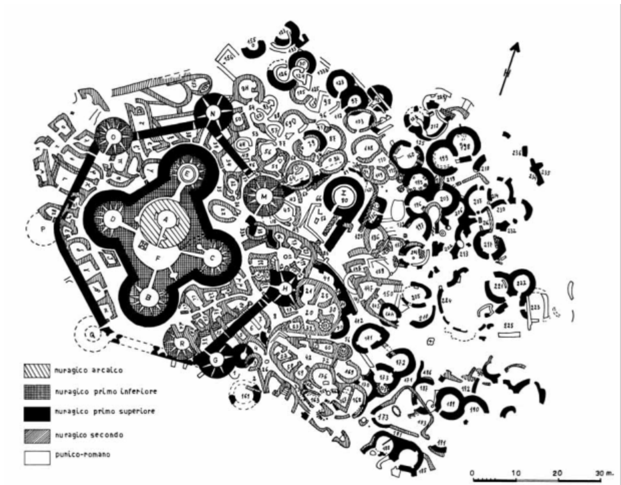
Fig. 1 - Planimetria del sito di Su Nuraxi, nuraghe e villaggio (da Lilliu 1962, Tavola LVI.1, p. 328).
