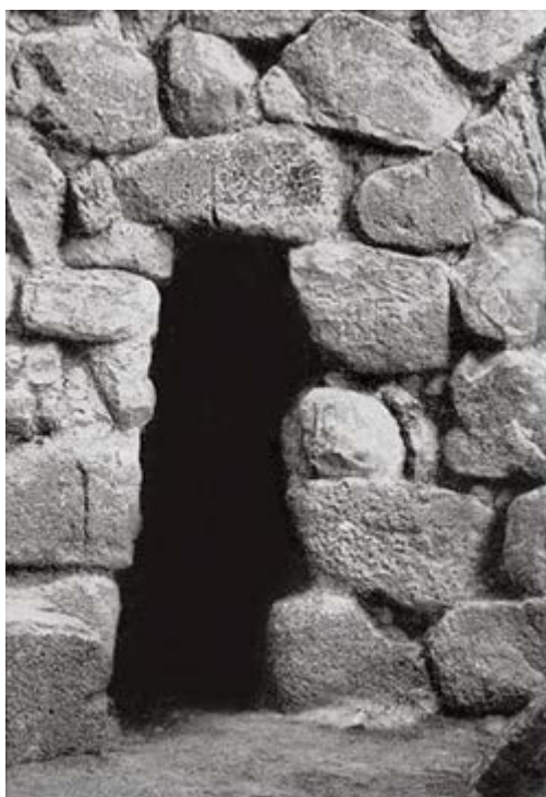
Fig. 2 - Porta d'ingresso alla torre B (da Lilliu 1962, Tavola LXIII.3, p. 335).
