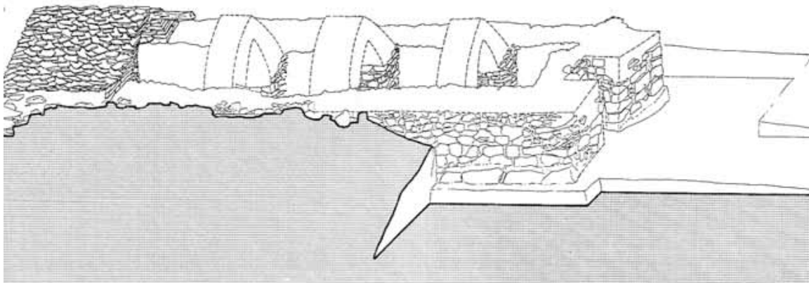
Fig. 3 - Ipotesi ricostruttiva della copertura del megaron 1 (da FADDA 2012, p. 13, fig. 14).
