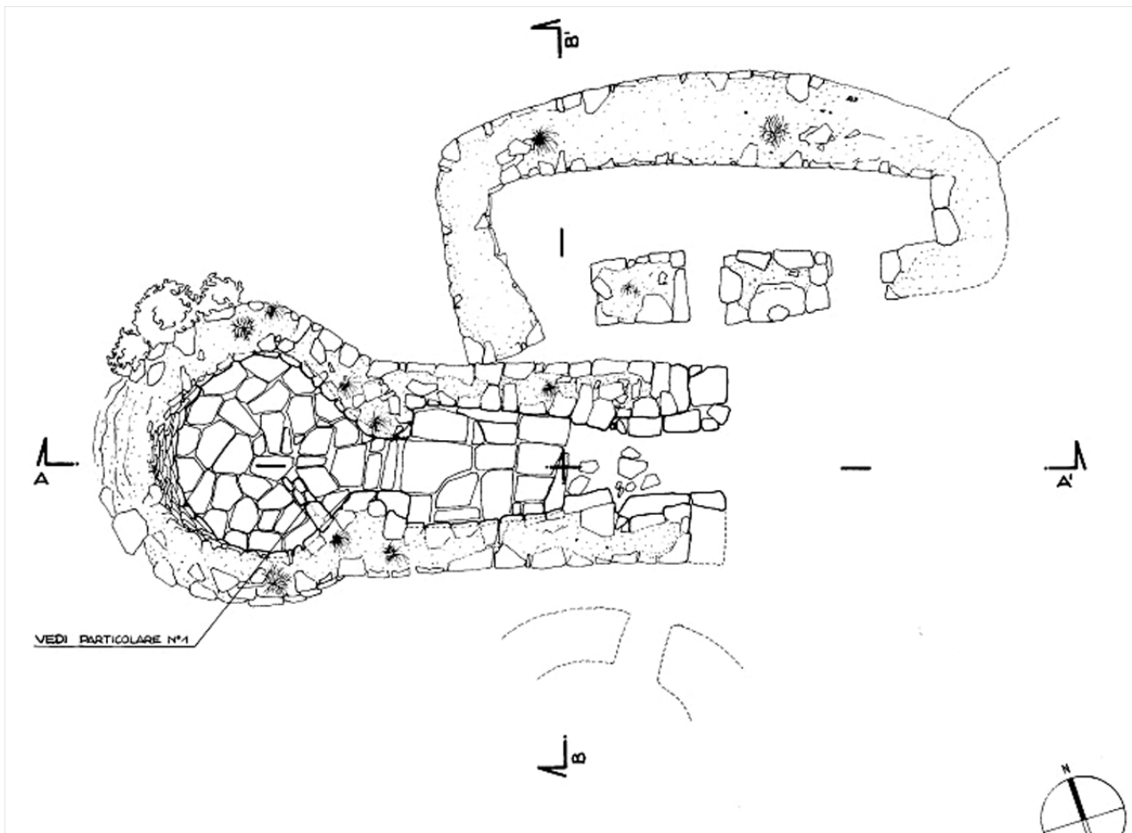
Fig. 1 - Planimetria del tempio di Sa Carcaredda (da FADDA 1995, p. 118, fig. 4.1).
