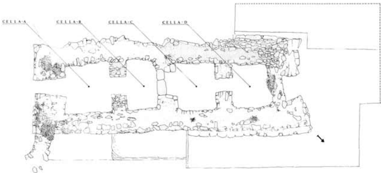
Fig. 1 - Planimetria tempio a megaron 1 (da FADDA 2012, fig. 9 p. 10).
