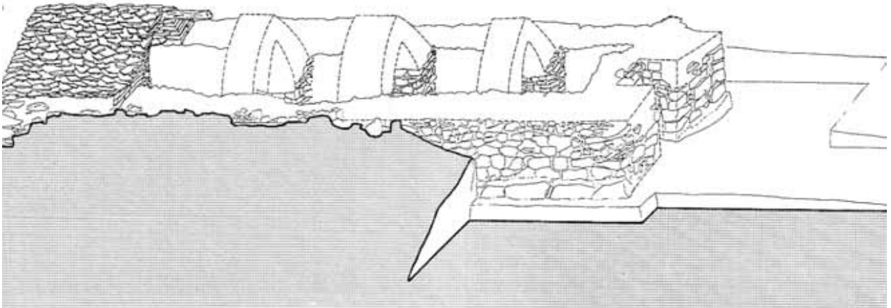
Fig. 2 - Ipotesi ricostruttiva della copertura a doppio spiovente del megaron 1 (da FADDA 2012, p. 13, fig. 14).
