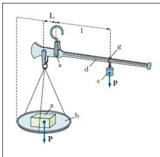
Fig. 3 - Il sistema di pesatura della stadera (da http://www.treccani.it/enciclopedia/stadera/ ).
