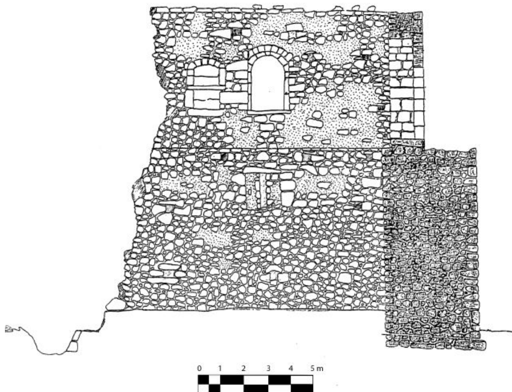
Fig. 4 - Luogosanto, Palazzo di Baldu: prospetto interno Ovest del Palazzo di Baldu (elaboraz. grafica di A. M. Azara).
