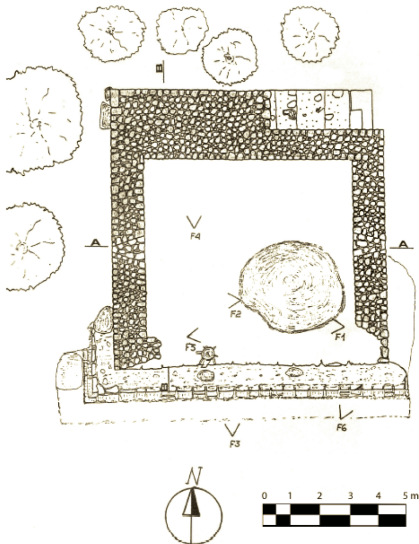
Fig. 1 - Pianta de Lu Palatzu (rilievo ed elaboraz. grafica di A. M. Azara).
