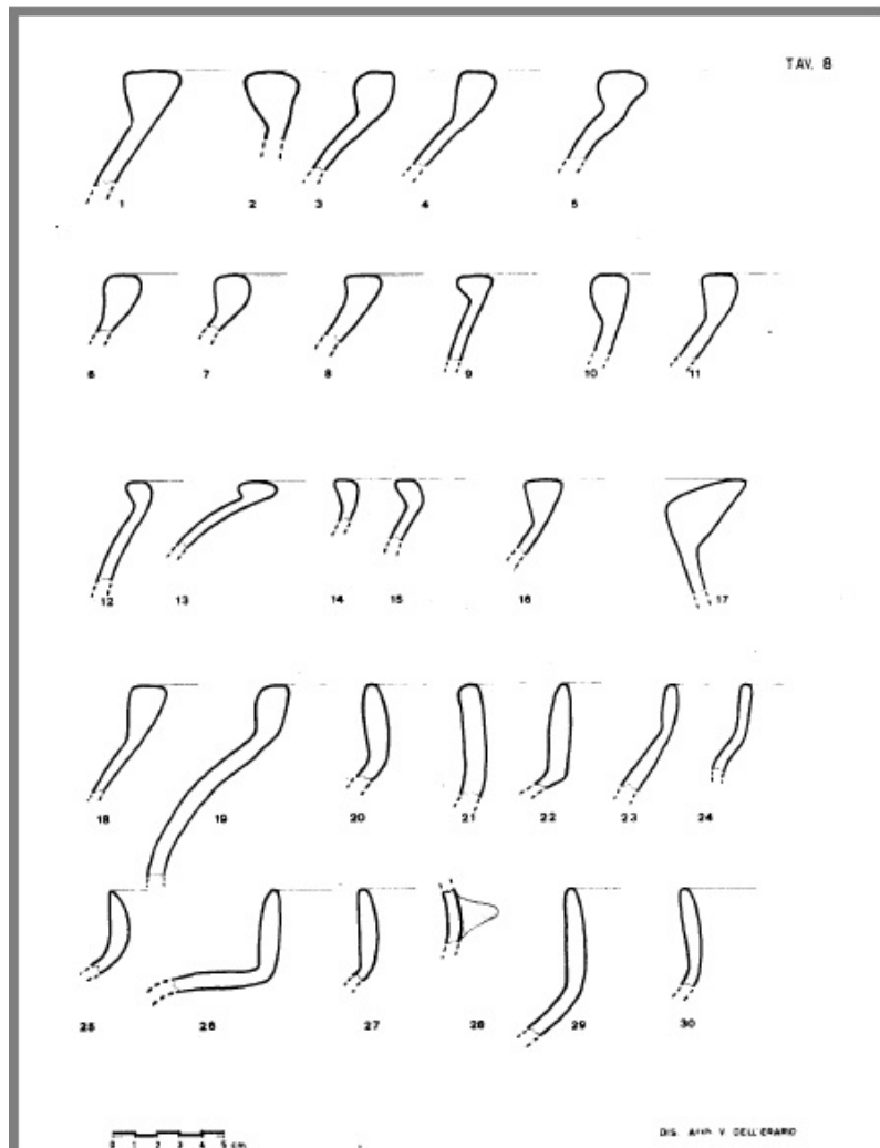
Fig. 1 - Diversi profili dell'orlo delle olle (da FADDA 1984, tav. 8).
