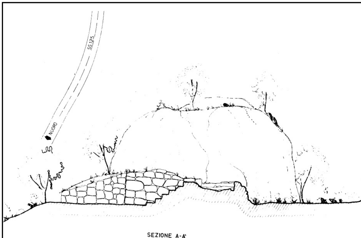
Fig. 3 - Sezione trasversale del nuraghe Monte Idda (da FADDA 1984, fig. 2).
