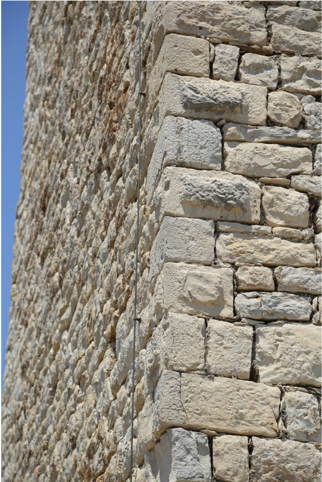
Fig. 3 - Conci impiegati negli angoli, alcuni dei quali lavorati a bugnato (foto di Unicity S.p.A.).
