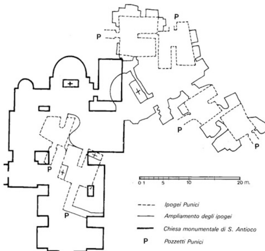
Fig. 4 - Pianta della Basilica di Sant'Antioco con Catacomba
