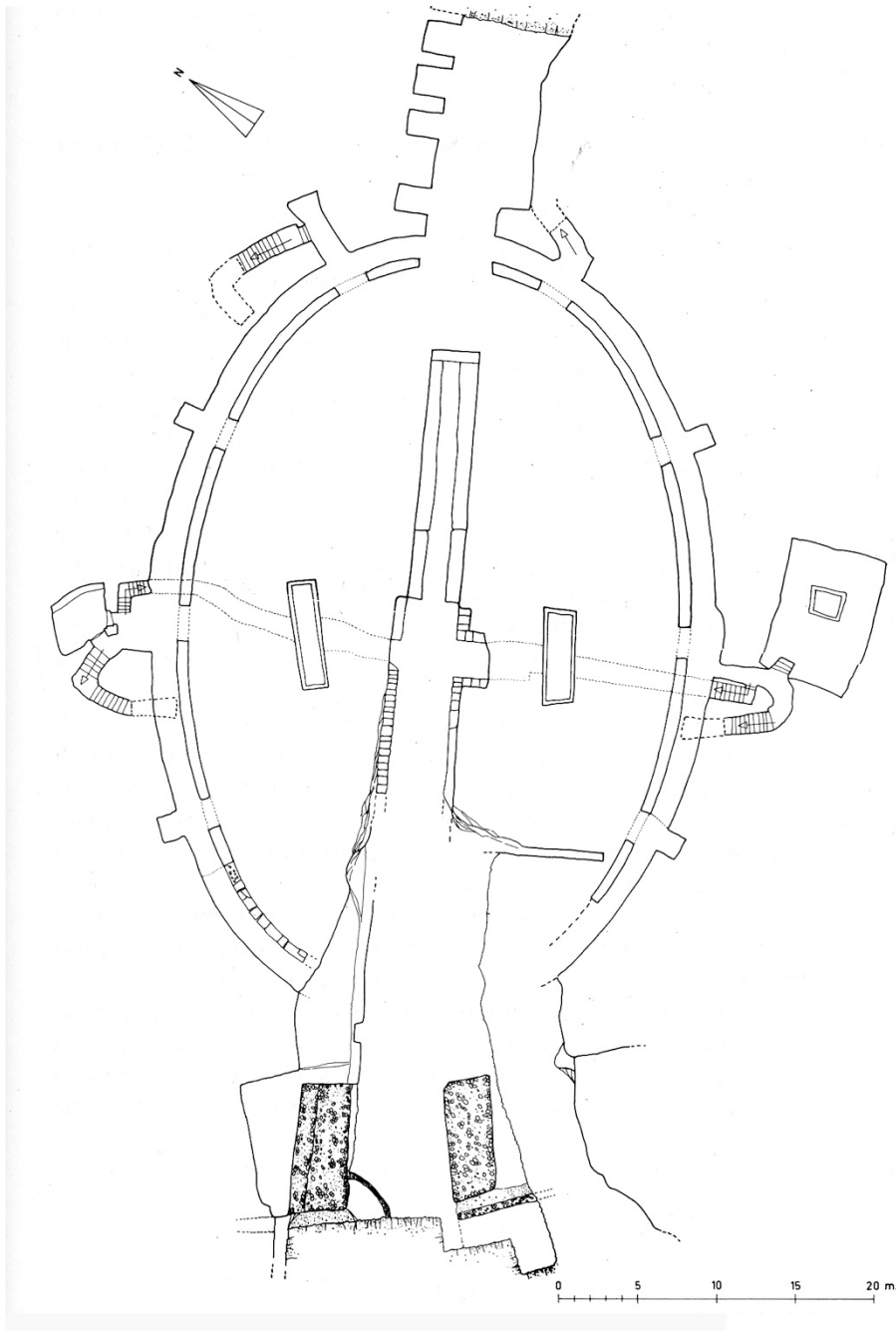
Fig. 4 - Pianta dell'anfiteatro romano di Cagliari (da PALA 1994, p. 147).
