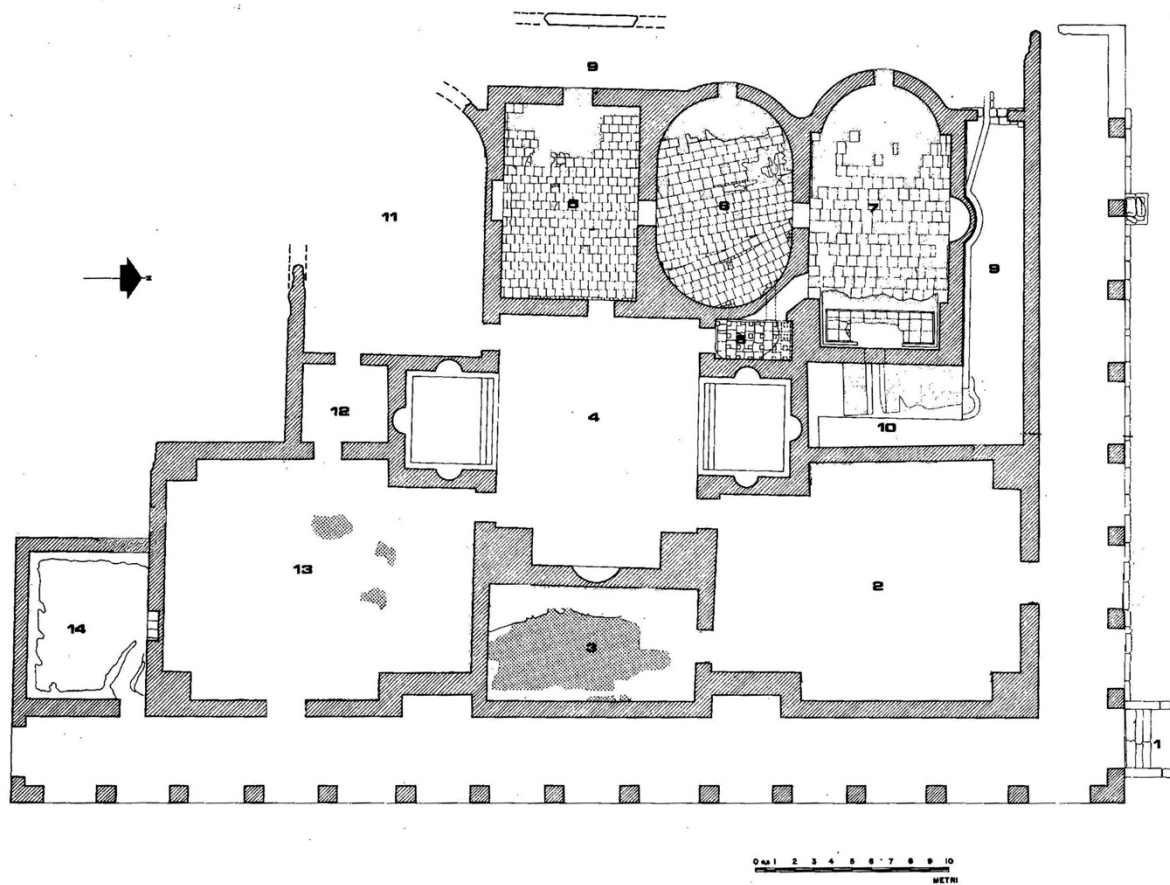
Fig. 2 - Le Terme a mare di Nora. Fase costruttiva degli inizi del III sec. d.C. (da TRONCHETTI 1985, fig. 12. Rielaborazione di C. Tronchetti)
