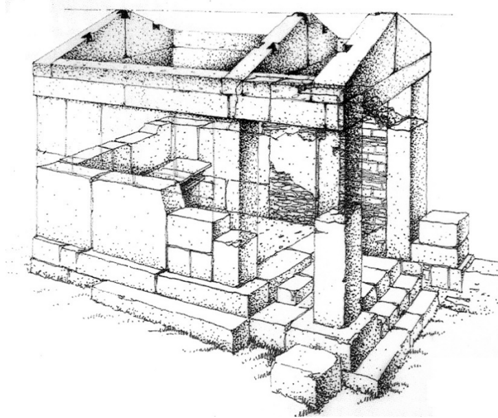
Fig. 4 - Ricostruzione del tempietto K (da ACQUARO 1988, p. 221)
