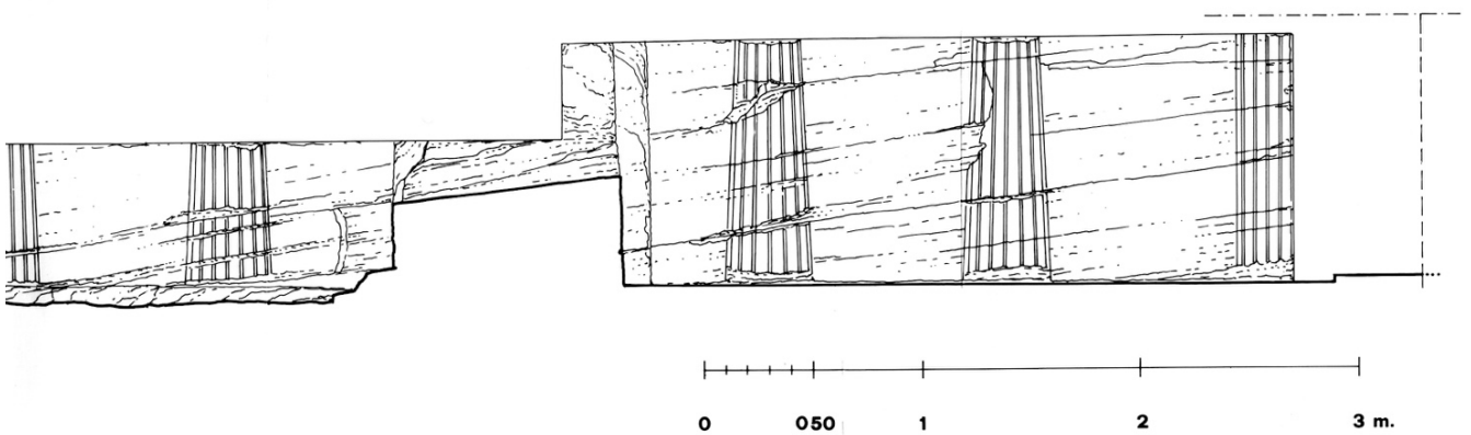
Fig. 7 - Rilievo del lato settentrionale del tempio delle semicolonne (da ACQUARO 1991, p. 541)
