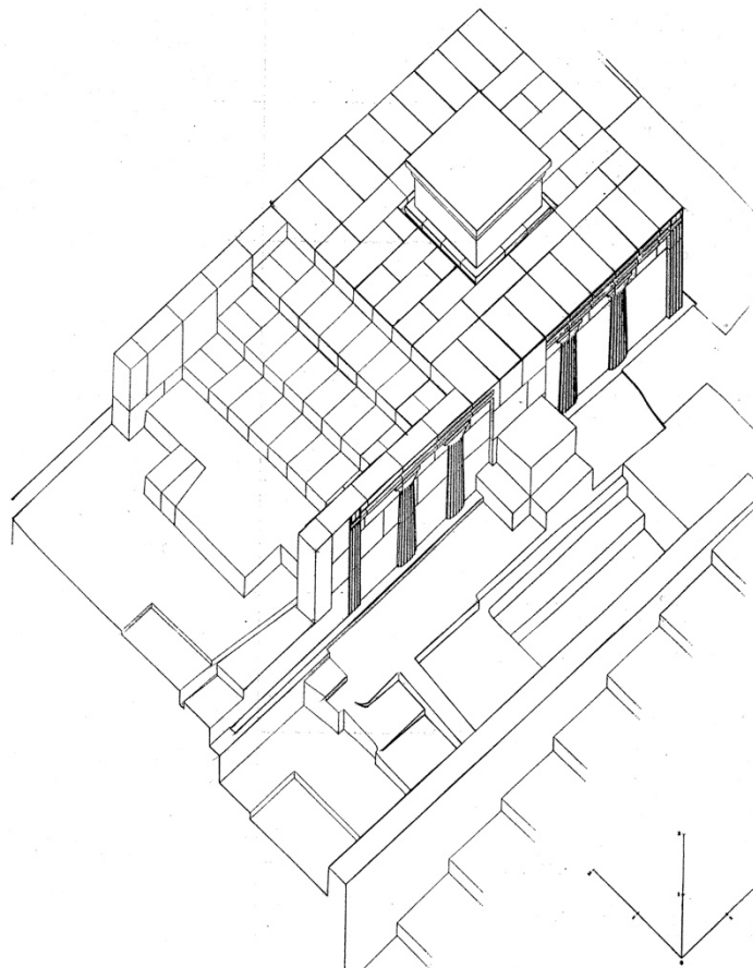
Fig. 8 - Assonometria ricostruttiva del tempio delle semicolonne (da PERRA 1998, p. 214)
