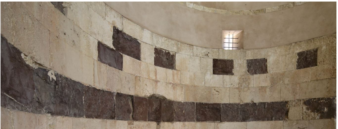
Fig. 3 - Détail de la technique de construction (photo Unicity S.p.A.).
