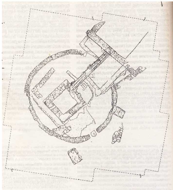
Fig. 2 - La place Sa Cosimo : planimétrie du puits (Pani Ermini, Spanu 1992, p. 26, fig. 16).
