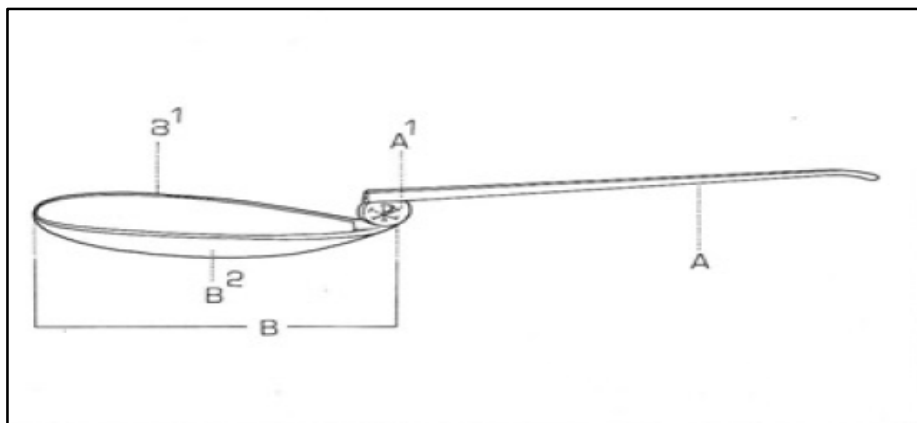
Fig. 4 - Petite cuiller liturgique : A - manche ; A1- raccord ; B - cuilleron ; B1- bord ; B2 - fond (MONTEVECCHI, VASCO ROCCA 1988, p. 143).
