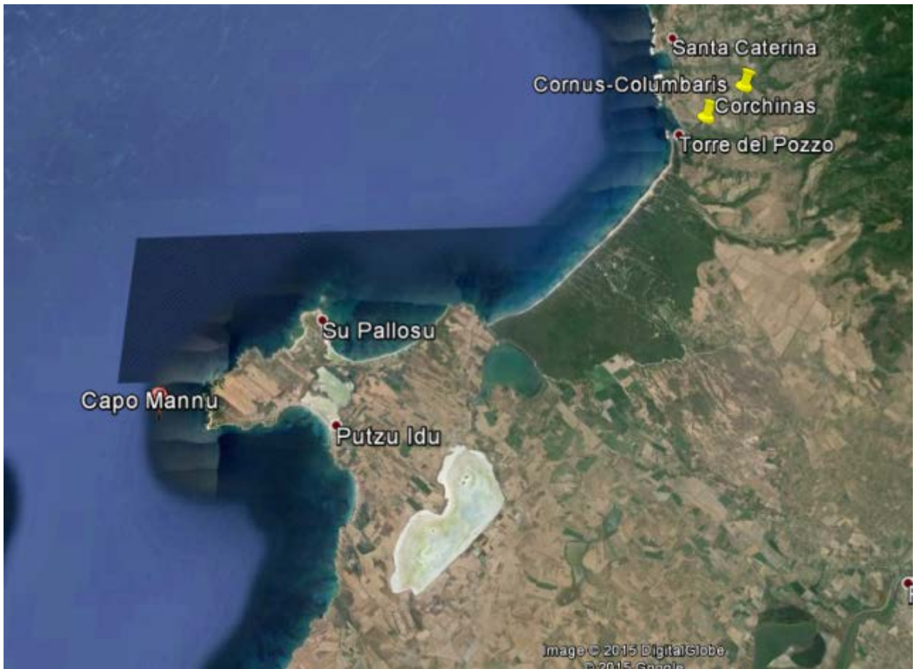
Fig. 3 - Image satellitaire Google Earth.
