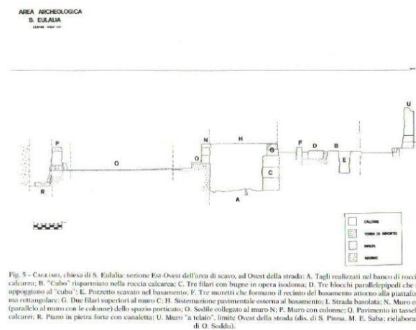
Fig. 2 - Section Est-Ouest de la zone occidentale de Sant'Eulalia (Martorelli et al. 2003, p.376, fig. 5).
