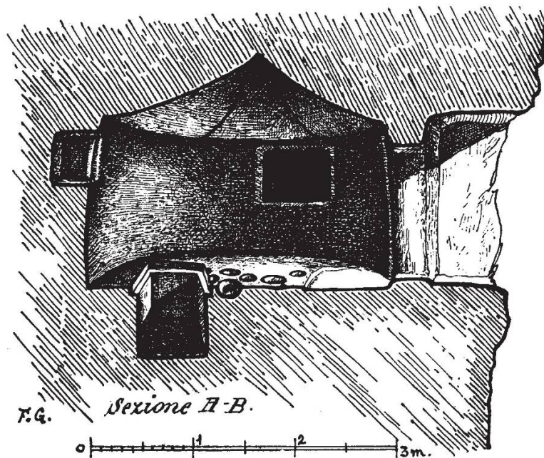
Fig. 3 - Section transversale de l'hypogée (Taramelli 1919, fig. 45, p. 103).
