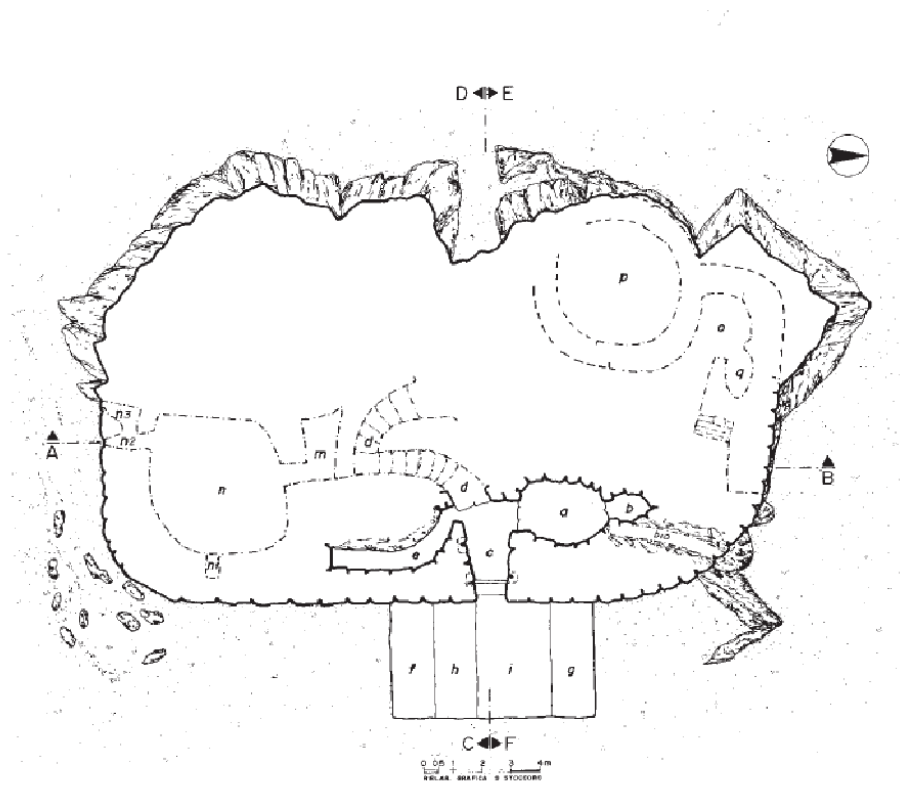
Fig. 1 - Nuraghe Albucciu, planimétrie du rez-de-chaussée (ANTONA-RUJU, FERRARESE CERUTI 1992, fig. 12).
