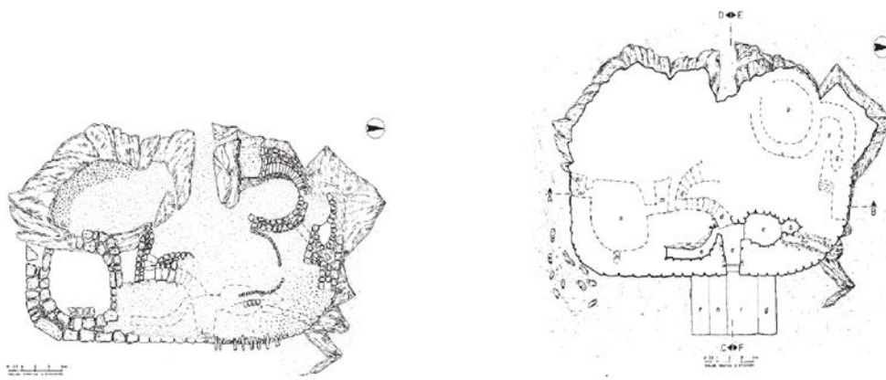
Fig. 1 - Nuraghe Albucciu, planimétrie du rez-de-chaussée et du premier étage (ANTONA-RUJU, FERRARESE CERUTI 1992, fig. 12).
