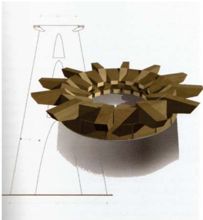
Fig. 1 - Représentation tridimensionnelle du système de la terrasse du donjon de Su Nuraxi (Cappai 2012, fig. 4, p. 35).
