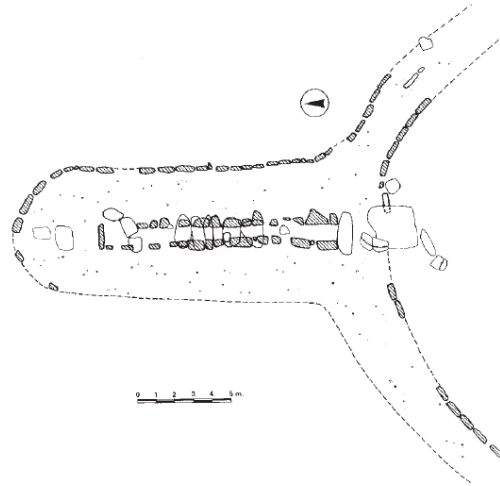
Fig. 1 - Planimétrie de la tombe des géants de type dolménique d'Abba Noa 1-Dorgali (MORAVETTI 1998, fig. 18, p. 27).
