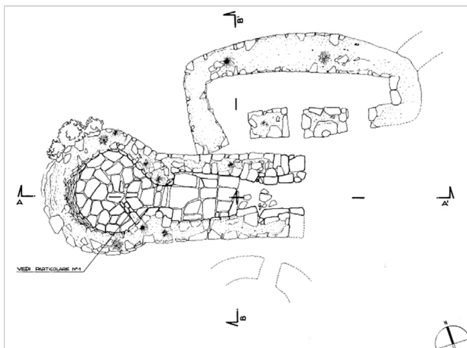
Fig. 1 - Planimétrie du temple de Sa Carcaredda (FADDA 1995, p. 118, fig. 4.1).
