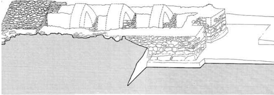
Fig. 2 - Hypothèse de reconstruction de la couverture à double pente du mégaron 1 (FADDA 2012, p. 13, fig. 14).
