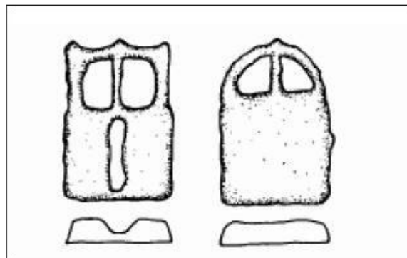
Fig. 2 - Dessin des lingots en étain de l'Époque Romaine provenant de l'épave de Port Vendres (PENHALLURICK 1986).
