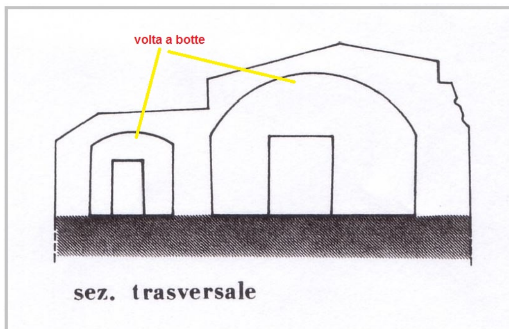
Fig. 4 - Section transversale du corps principal (réélaboration de M. G. Arru à partir de Zucca 1987, pl. 27, p. 258).
