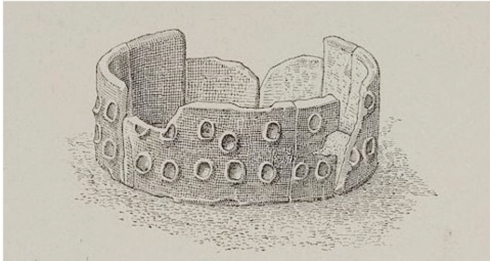
Fig. 2 - Reconstruction graphique du soi-disant four de fusion identifié par A. Taramelli (Taramelli 1918, coll. 115-116, fig. 114).
