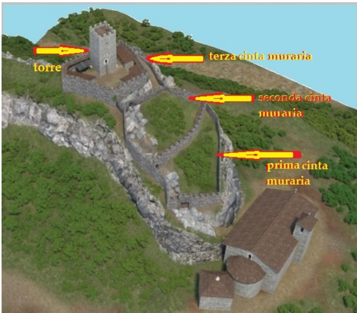
Fig. 2 - Reconstruction du château de la Fava avec l'indication des murs d'enceinte (réélaboration de M. G. Arru, reconstruction d'Unicity S.p.A.).
