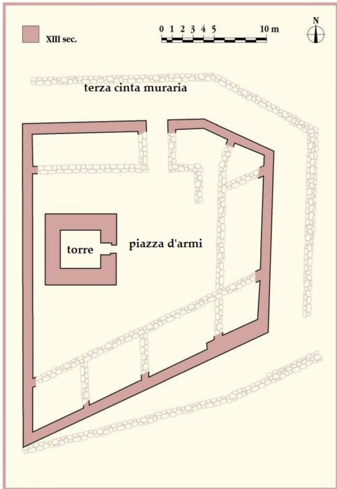
Fig. 5 - Plan du château de la Fava, Posada (CORONEO 1993, fiche 177, p. 295)
