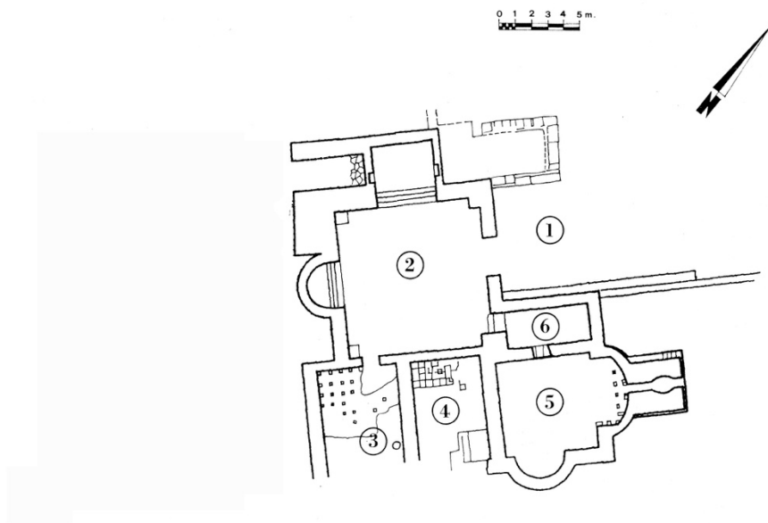
Fig. 5 - Planimétrie des Thermes : 1) apodyterium , 2) frigidarium , 3-5) calidaria , 6) passage (ZUCCA 1984, p. 85)
