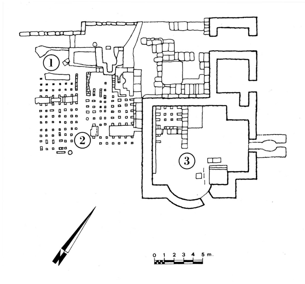
Fig. 3 - Plans des Thermes n°1 : 1) vestiaires ; 2) calidarium ; 3) calidarium (ZUCCA 1984, p. 88)
