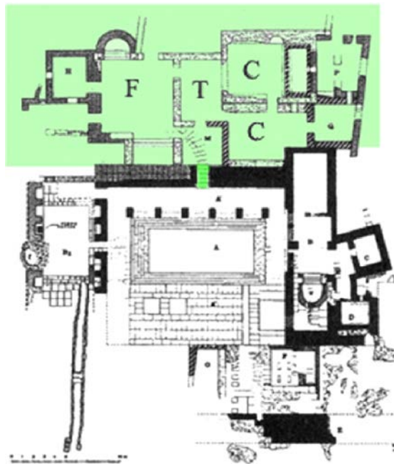
Fig. 1 - Les Thermes II : le nouveau bâtiment est indiqué en vert et on signale la fonction des salles : F = frigidarium ; T = tepidarium ; C = calidarium (Bacco, Serra 1998, p. 1220, réélaboration de C. Tronchetti).
