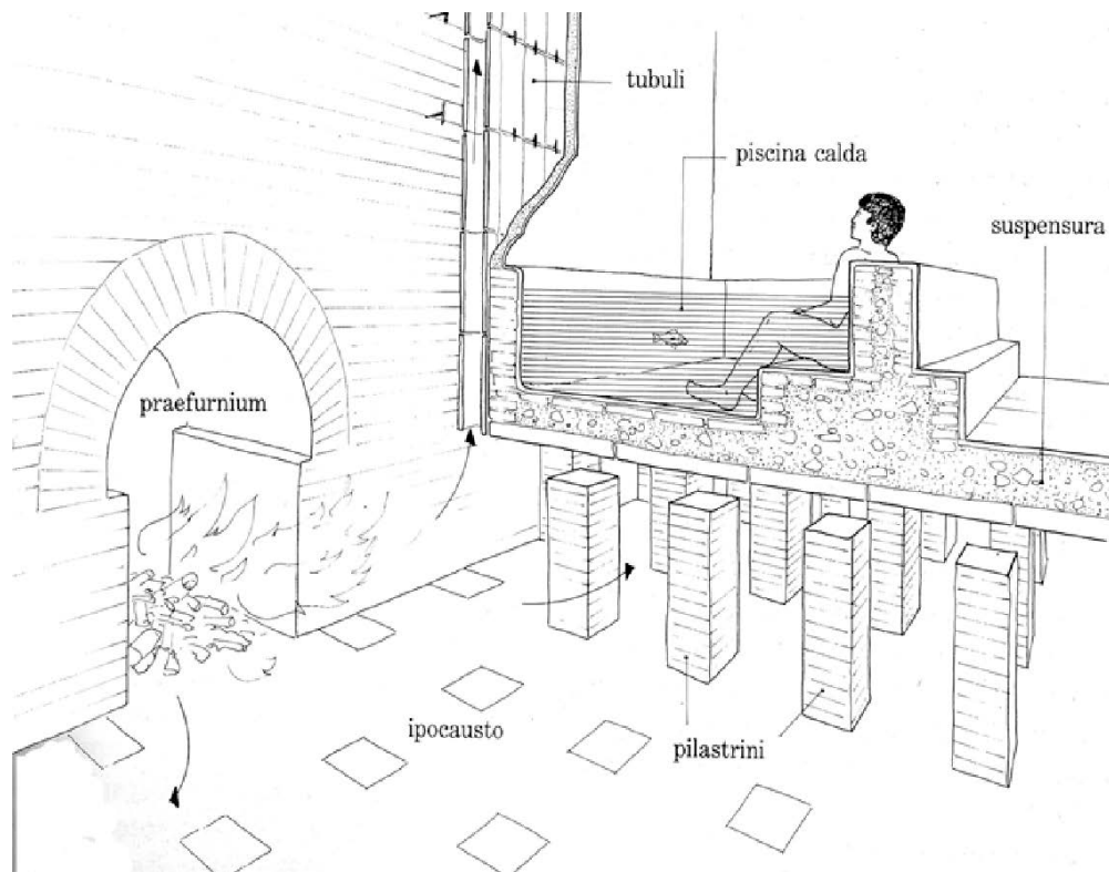
Fig. 2 - Système de chauffage des locaux : l'air chaud provenant du four pénétrait sous le sol soutenu par des suspensurae et, en passant à travers les tubuli percés à l'intérieur des murs, il créait une isolation chaude de la pièce (Adam 1988, p. 293).
