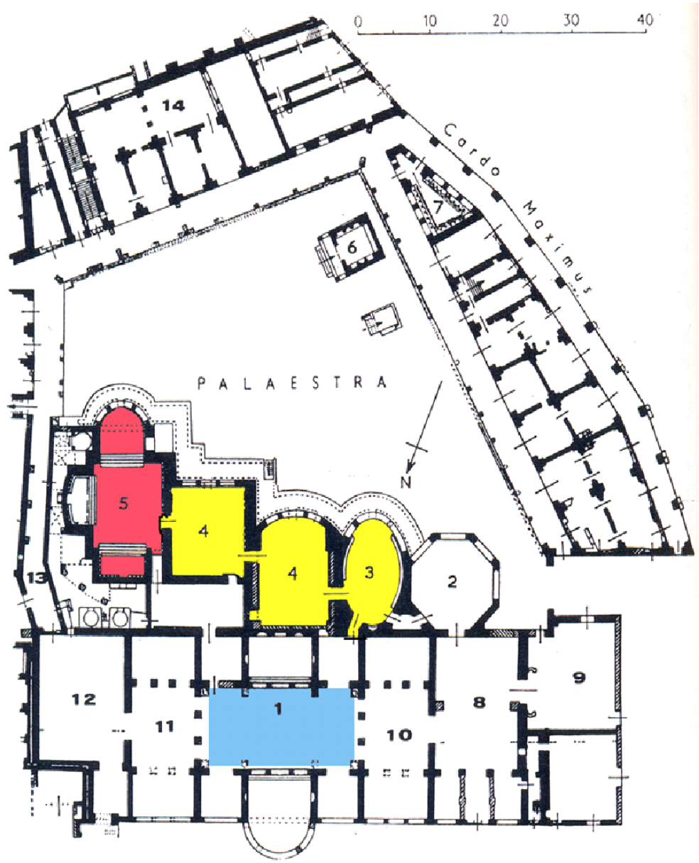
Fig. 1 - Ostie, Thermes du Forum (II e siècle ap. J.-C.). Les salles des thermes : le frigidarium indiqué en bleu ciel ; le tepidaria en jaune et le calidarium en rouge (Pavolini 1983, réélaboration de C. Tronchetti).
