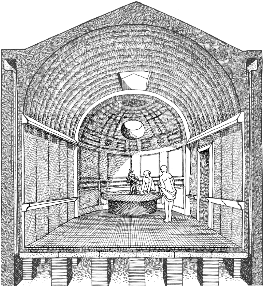
Fig. 4 - La reconstruction illustre l'abside d'un calidarium avec une cuvette d'eau pour se rafraîchir. On y découvre le système de chauffage de la salle ( suspensurae ) et l'éclairage assuré par des fenêtres et des lucarnes (Macaulay 1978, p. 86).
