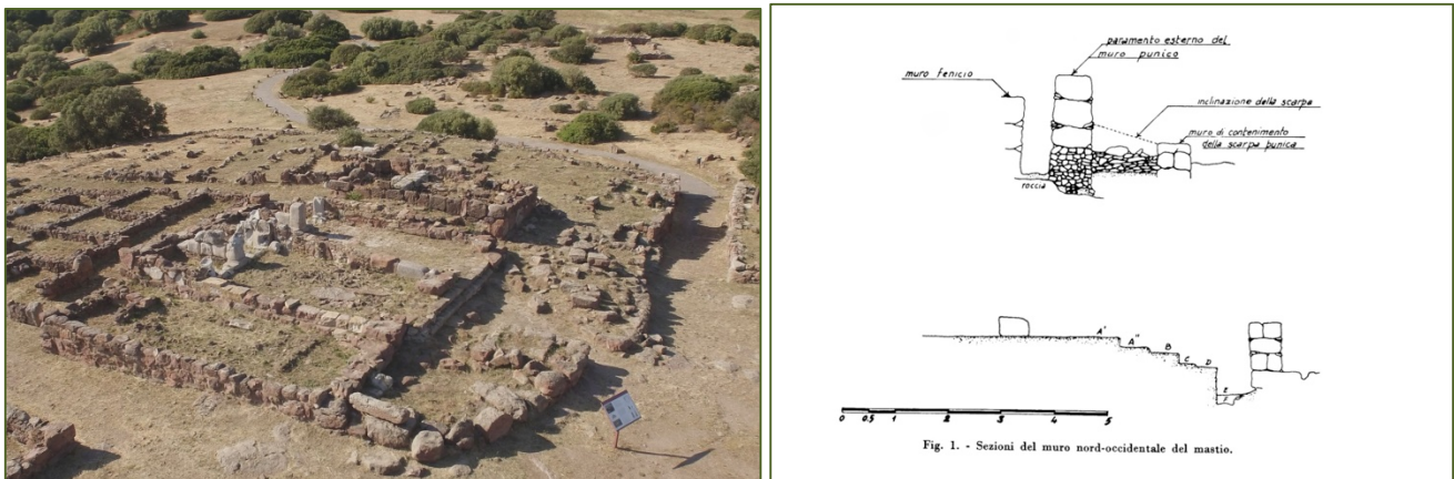
Fig. 1, 2 - Le « temple d'Astarte » (photo Unicity S.p.A.) ; une stratigraphie des fouilles 1966 (MONTE SIRAI - IV, fig. 1).
