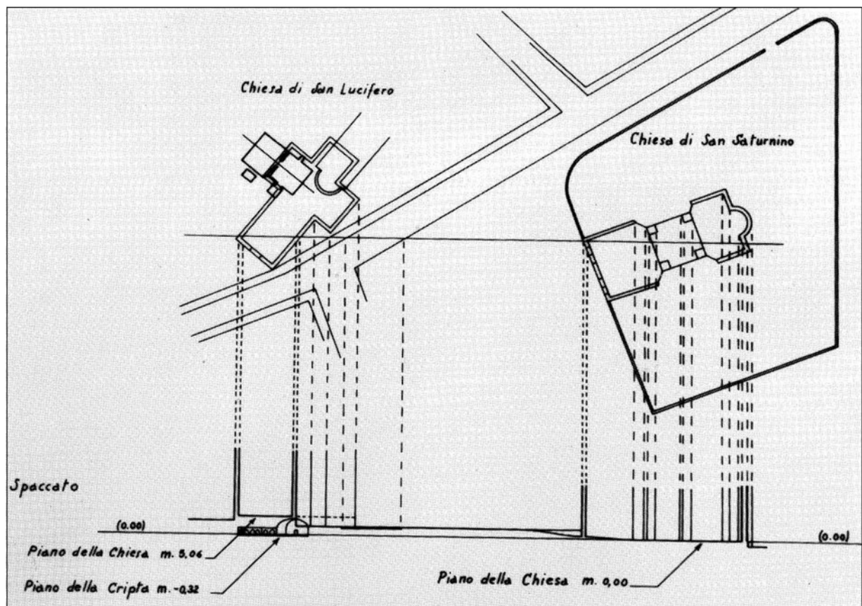
Fig. 1 - Planimetría de los ambientes subyacentes de la iglesia de S. Lucifer en relación con la basílica de S. Saturnino (de Mureddu et alii 1988, p. 156, lám. 12).
