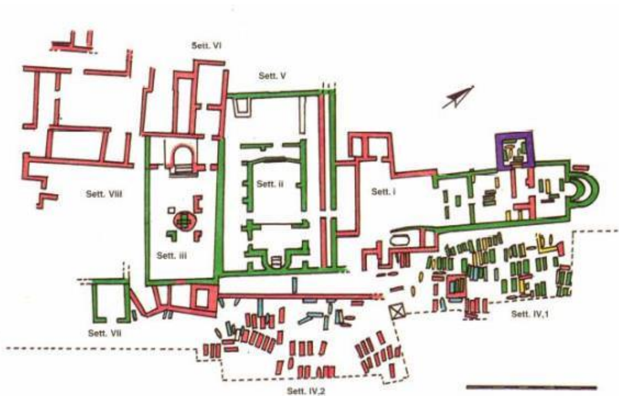
Fig. 3 - Planimetría del complejo de Columbaris-Cornus donde se indican las fases y los sectores (elaboración gráfica de L. SALADINO, M. C. SOMMA, de Cornus I.1, pág. 200, lám. II).
