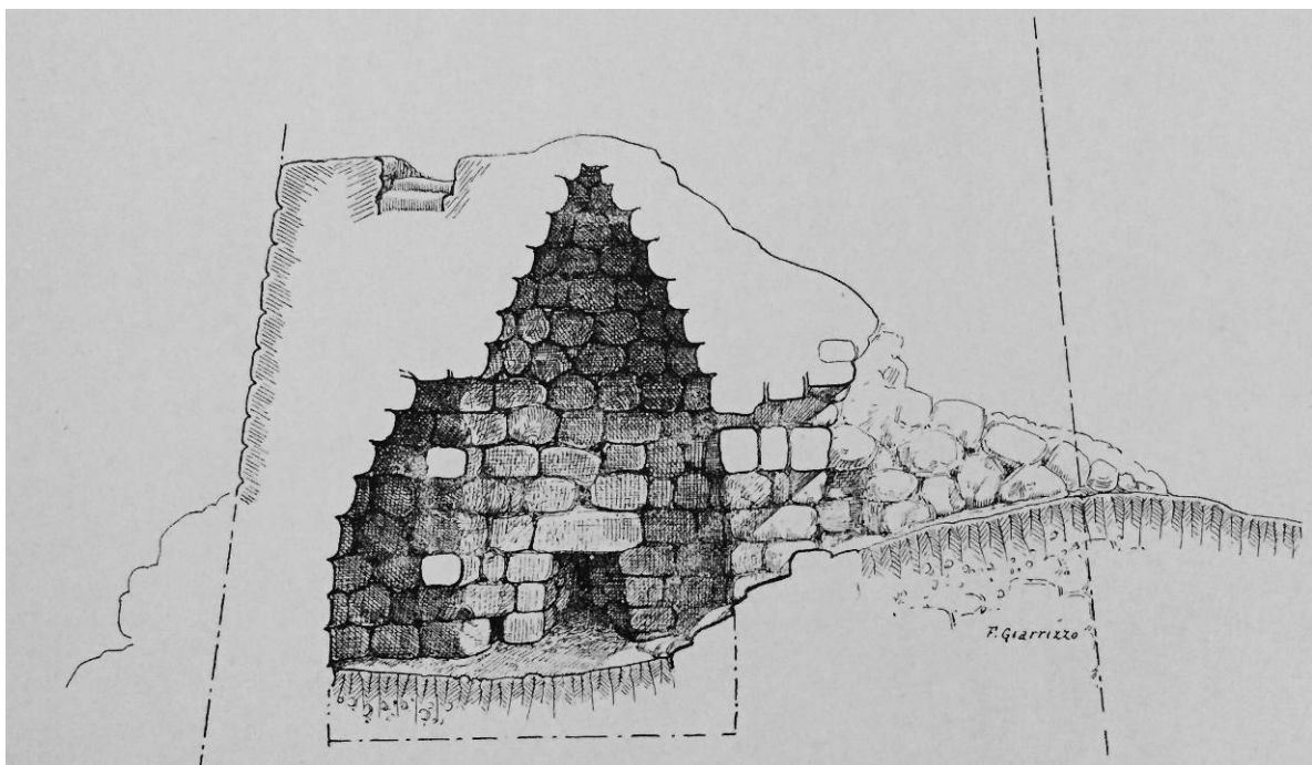
Fig. 1 - Sección del nuraga Puttu de Inza (de Taramelli 1919, fig. 30, págs. 73 - 74).
