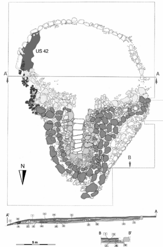
Fig. 3 - Planimetría de la tumba de los gigantes de Pala'e Sulzaga-Bonorva (de Ialongo, Usai, Vanzetti 2012, fig. 2, pág.1453).
