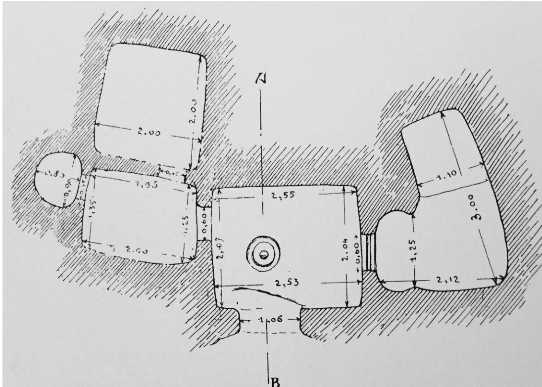
Fig. 3 - Planimetría de la domus de janas XIII (de Taramelli 1919, fig. 57, págs. 119, 120).
