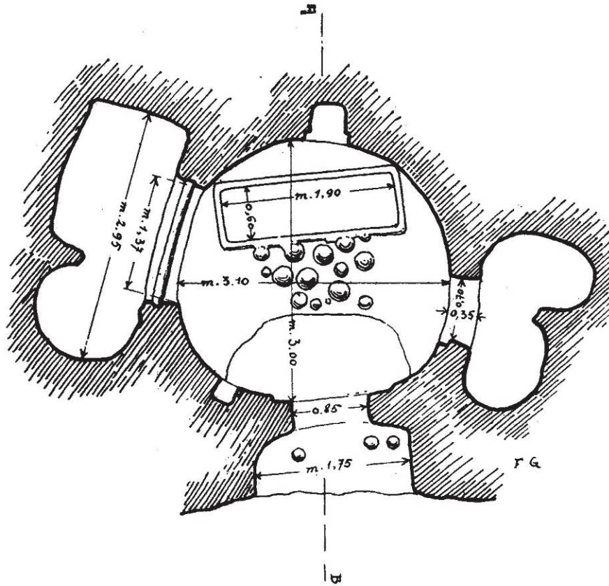
Fig. 2 - Planimetría de la domus de janas (de Taramelli 1919, fig. 44, pág. 102).
